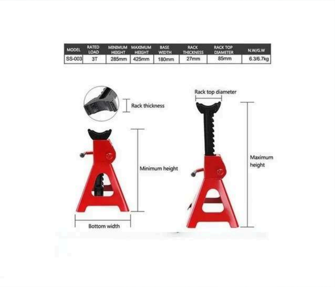
SET 2 BANQUILLO MECÁNICO 3 TON CABALLETE SOPORTA GATA HIDRÁULICA
